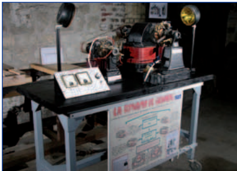
La dynamo de Gramme est bidirectionnelle : alimentée en électricité, elle produit une force mécanique, alimentée en énergie mécanique, elle produit du courant continu.
